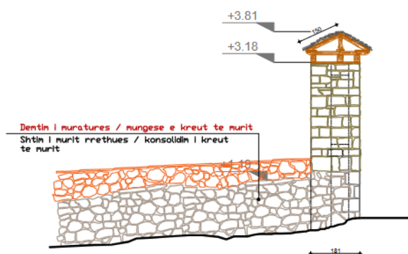
PAMJA JUGORE
