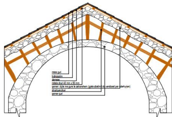
DETAJ I KUNETES
