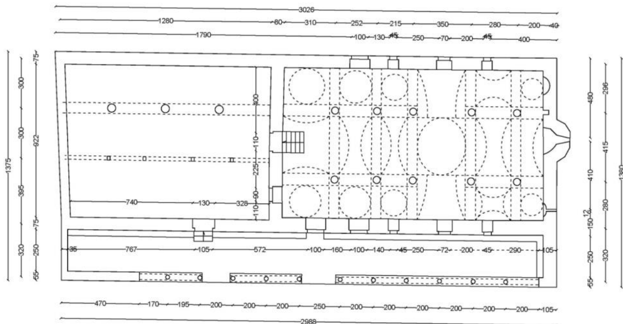
Plani I Kishës (Skicat referuar projektit të miratuar në vitin 2008)
