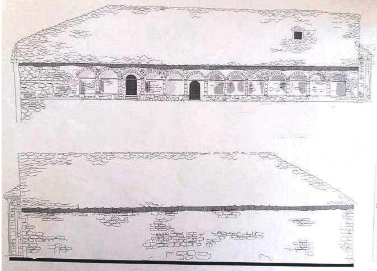
Fasada Jugore dhe Veriore (Skicat referuar projektit të miratuar në vitin 2008)
