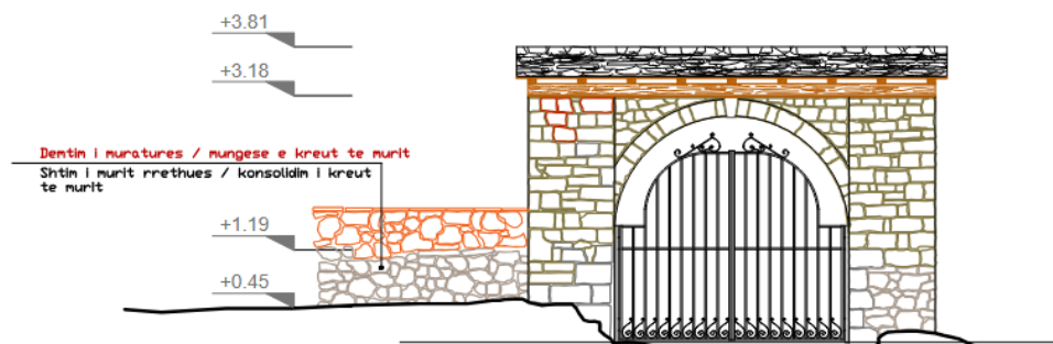
PAMJA PERENDIMORE
