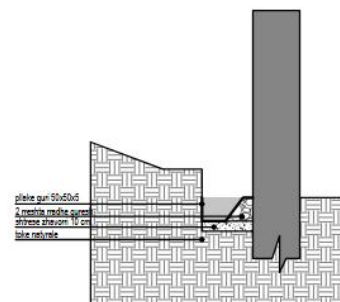
DETAJ I KUNETES
