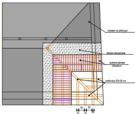
DETAJ I CATISE
